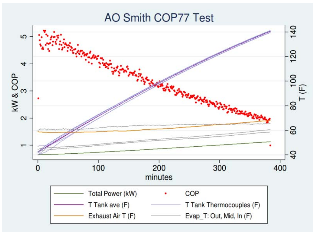
B 10. AO Smith Voltex COP77 Test
