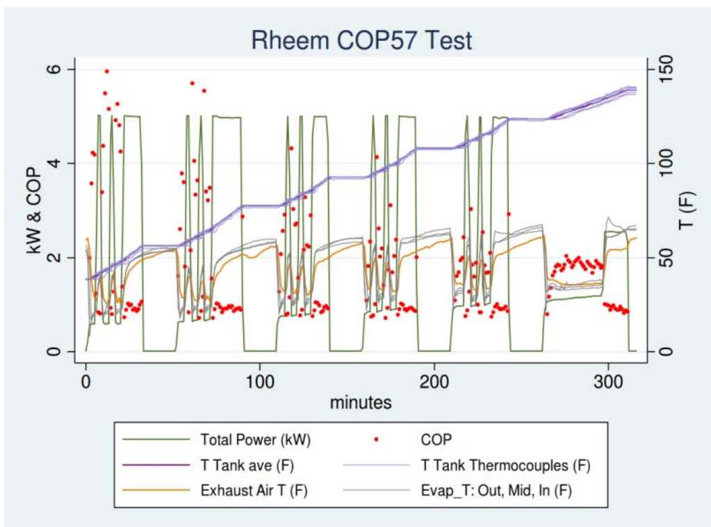
B 6. Rheem EcoSense COP57 Test
