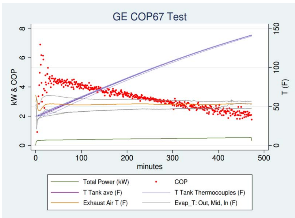
B 8. GE GeoSpring COP67 Test
